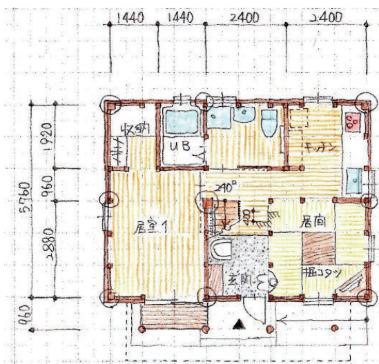
【平面プラン】
