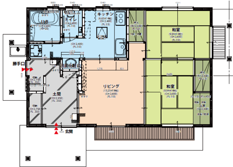
【平面プラン】
